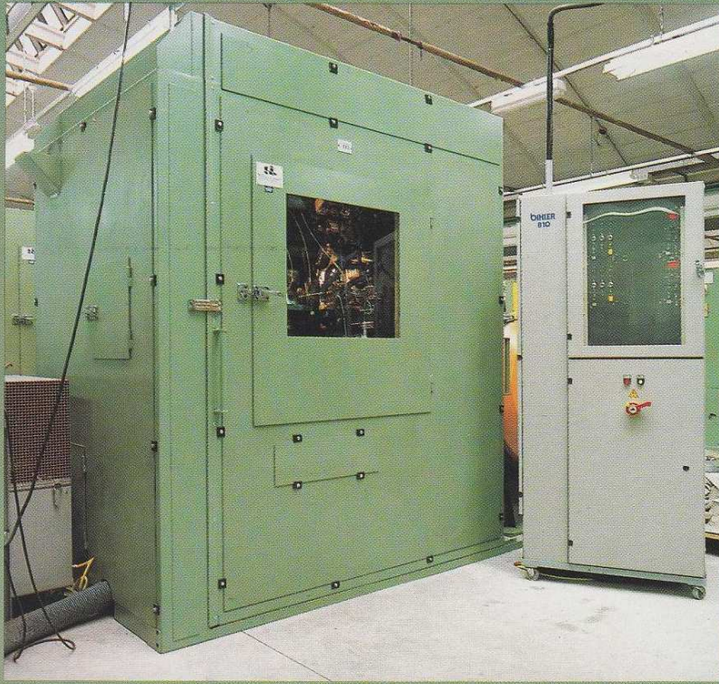
Cabina di insonorizzazione scorrevole su macchina pressopiegatrice.
